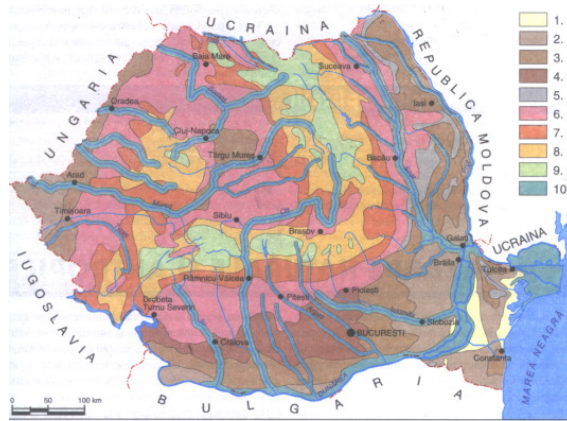
Soluțiile Române (1. soluri baltane; 2. cernoziomuri; 3. cernoziomuri levigate; 4. soluri brun roșcate; 5. soluri cenușii; 6. soluri brune-lujvice; 7. soluri eu-mezobazice; 8. soluri brun acide;
